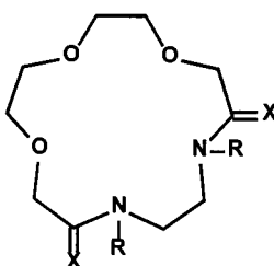
8a X=H 2 ; R=H 8b X=H 2 ; R=Me 11 8c X=O; R=H ~8
