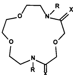
7a X=H 2 ; R=Me 21 7b X=O; R=H
