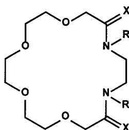
5a X=H 2 ; R=R'=H 15 5b X=H 2 ; R=R'=Me 27 5c X=O; R=R'=H
