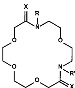
4a X=H 2 ; R=R'=H 24 4b X=H 2 ; R=R'=Me 28 4c X=O; R=R'=H 12
